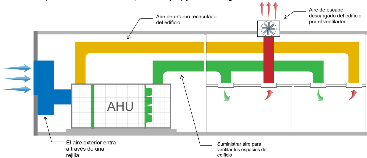
Figura 1. Esquema del sistema de ventilación.
