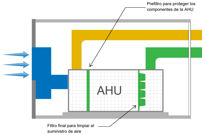
Figura 2. Lugares del filtro previo y final.
